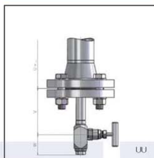
Фланцевое соединение EN/ANSI со сливным игольча- тым вентилем
