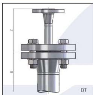
Фланцевое соединение EN/ANSI с вентиляционным фланцем
