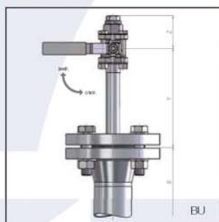
Фланцевое соединение EN/ANSI с вентиляционным шаровым вентилем
